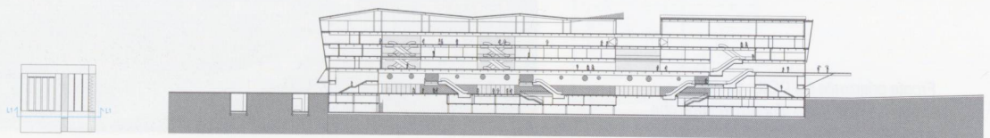
Sezione longitudinale
