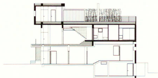
Sezioni
