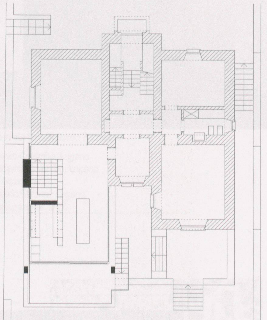
Pianta piano rialzato prima e dopo l'intervento
