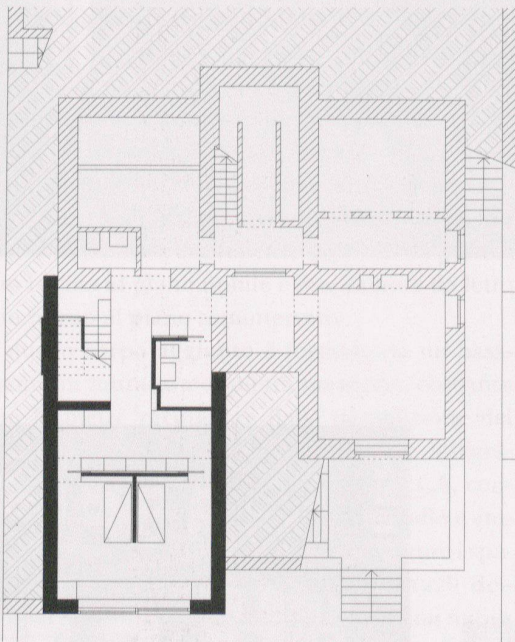
Pianta piano seminterrato prima e dopo l'intervento
