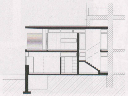
Sezione
