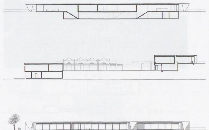
Sezioni
