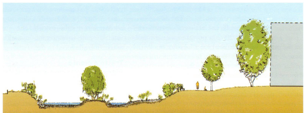
Sezione A-A sull'ansa del fiume, in cui appare l'allargamento dell'alveo che ha permesso la formazione di una penisola, parte della più ampia area naturalistica, delimitata dal percorso pedonale. ➔
