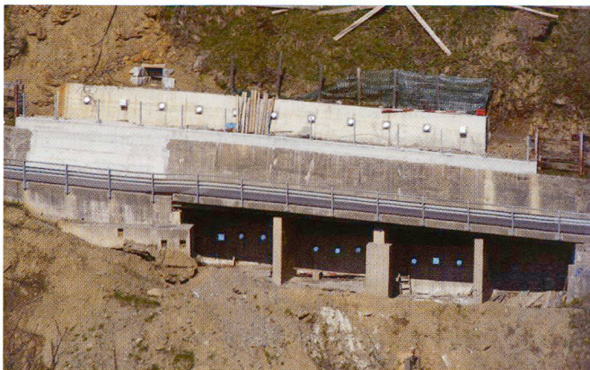
Intervento specialistico. Consolidamento pendio
