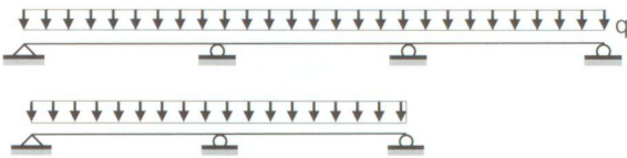
Modifica del sistema statico durante la demolizione
