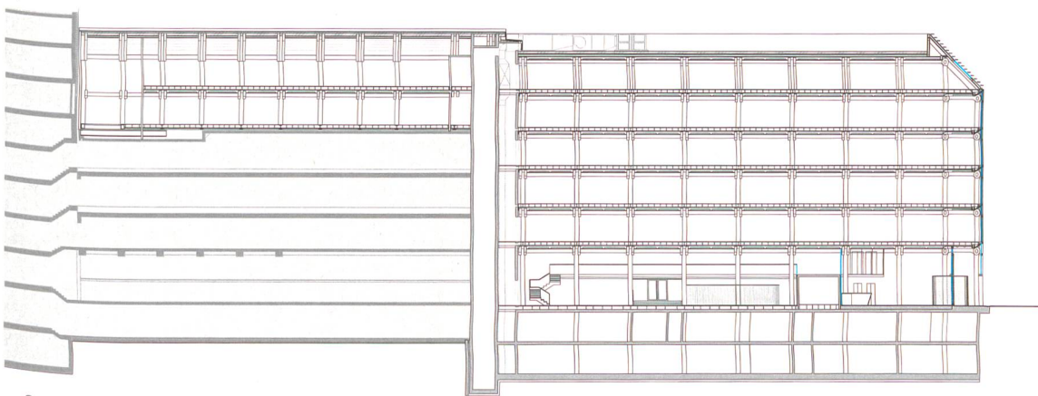
Sezione longitudinale
