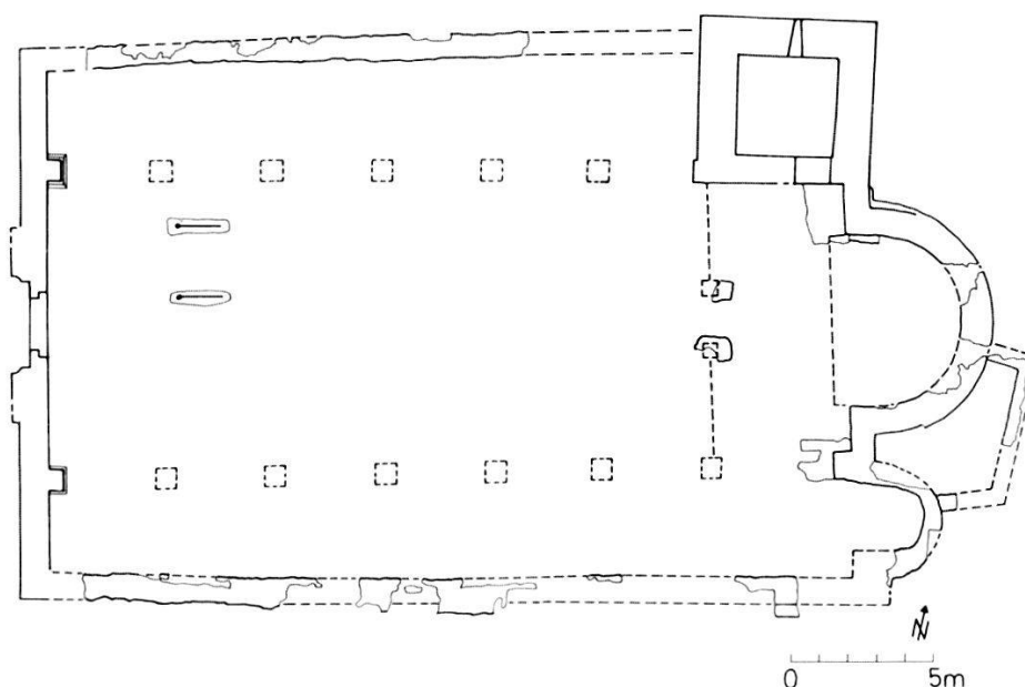
Abb. 6: Grundriss Bauphasen 6 – 7
