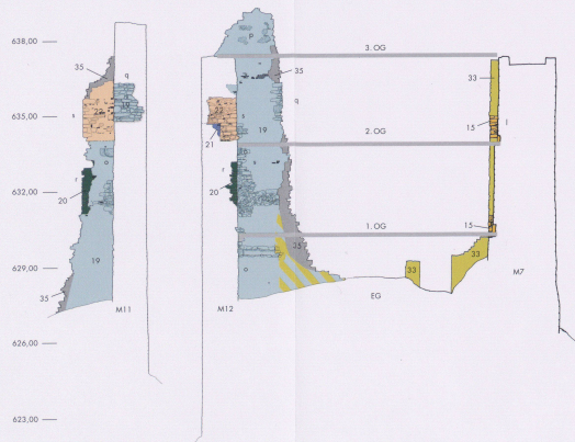
55 Palas, Schnitt von Osten, Mauer M12 von Norden (KAAG)
