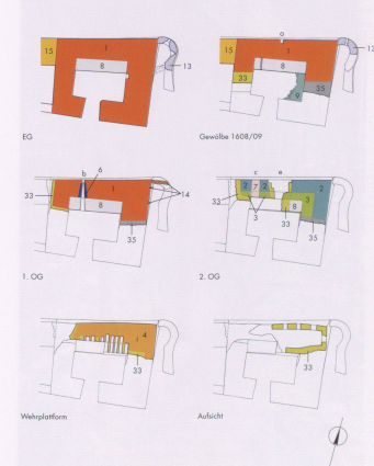
54 Hauptturm Gewölbeansicht (KAAG)
