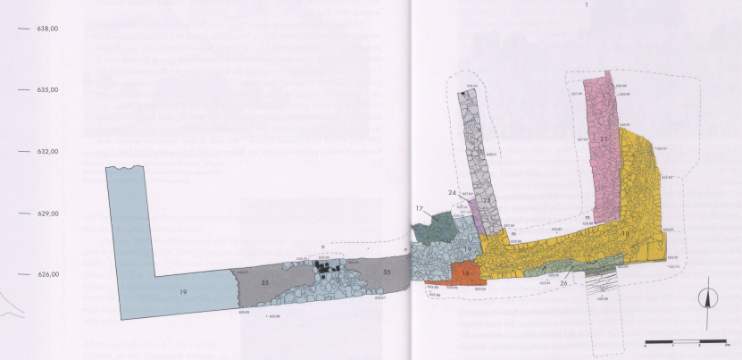
57 Palas Südteil, Aufsicht (KAAG)
