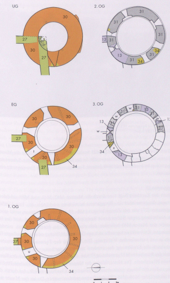
61 «Geisturm» - Rundurm M47, Geschossgrundrisse (KAAG).
