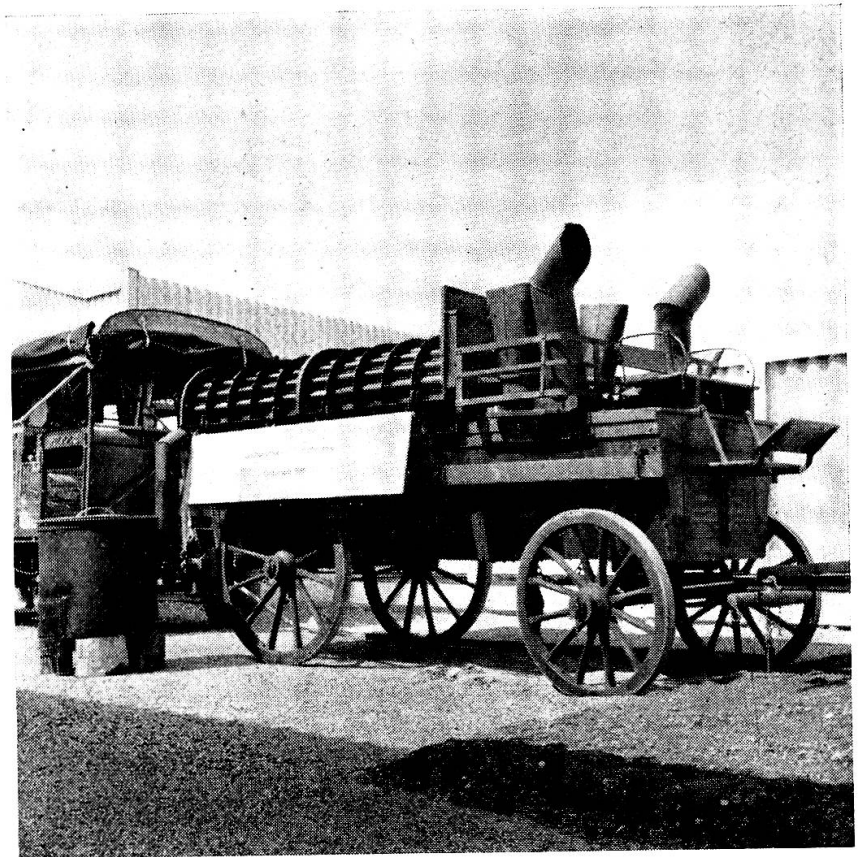
Gerätschaftswagen für eine Feldbäckerei, Ord. 1885
