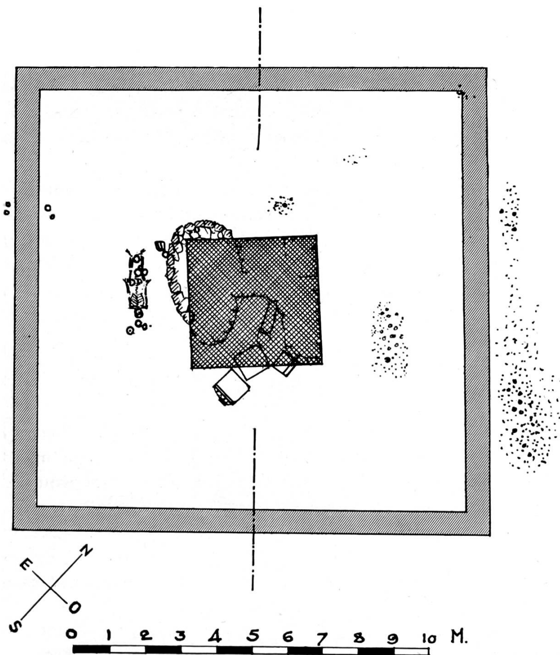
Fig. 23. Wavre, Mausolée romain. Plan général.
