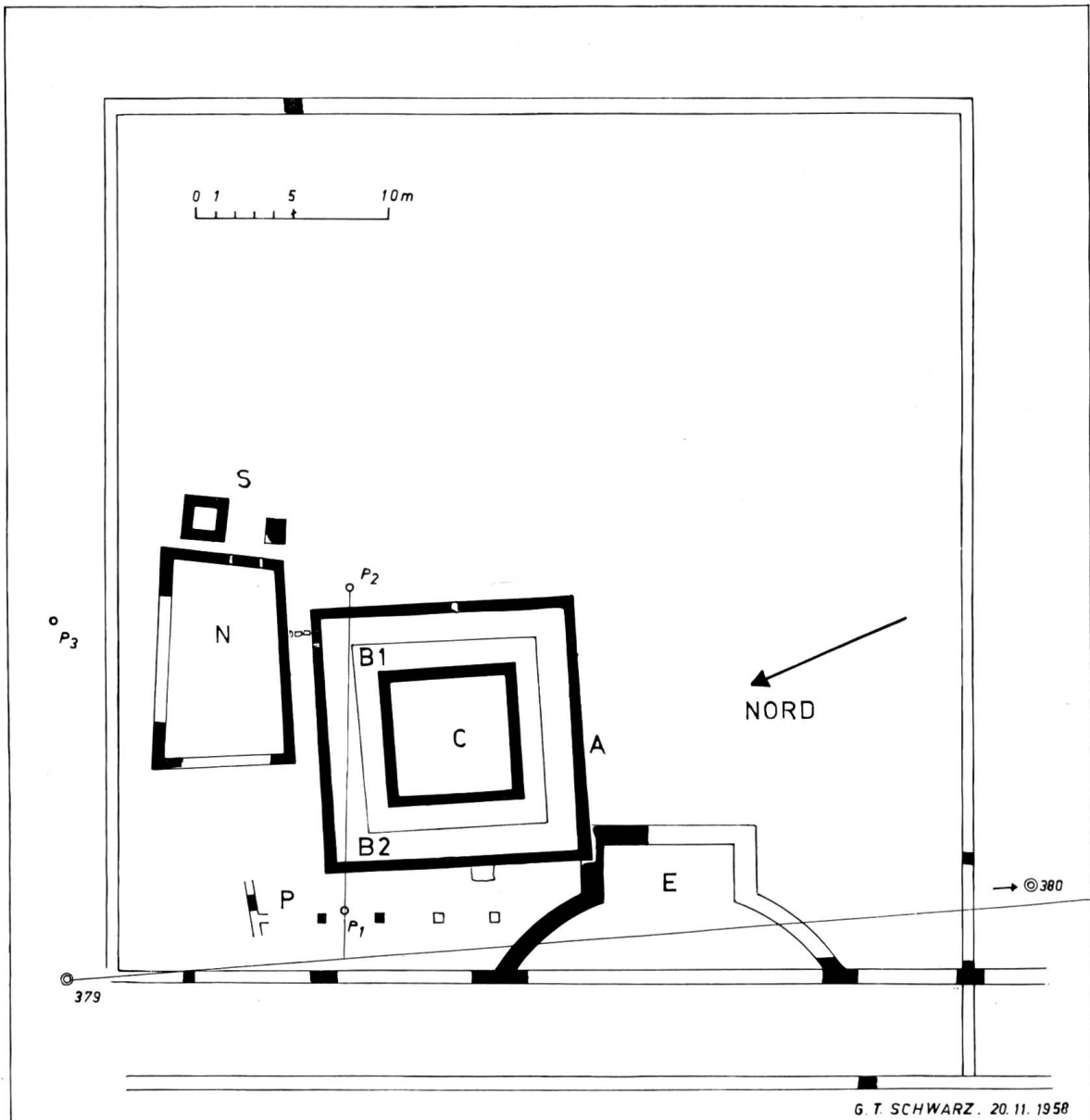
Abb. 3. Augst, Sichel. Gallorömischer Tempel, Grundriß. – Legende: A = Außenmauer; B 1 = Mörtelboden, Bauperiode I; B2 = Mörtelboden II; C = Cella; E = nischenartige Erweiterung in der Hofmauer; N = Nebengebäude (Priesterhaus?); P = Porticus; p 1, 2, 3 = Meßpunkte; S = gemauerte Sockel.
