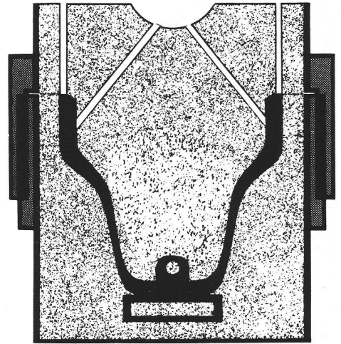
Abb. 13 Moderne Sandgussform für Kuhglocken: oben Gussdelle (mit zwei Gusskanälen) und zwei seitliche Luftkanäle. Nach M. Fonjallaz (wie Anm. 4). Forme en sable moderne pour la fabrication de cloches de vaches. Forma di sabbia moderna per la fabbricazione di campane per mucche.
