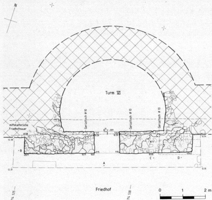
Grundriss des Mauerturmes VI. Plan de la tour VI. Pianta della torre VI.
