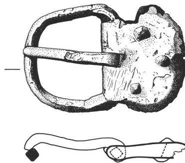
Abb. 4 Bronzeschnalle mit flachovalem Beschläg. Zeichnung M. 1:1. Boucle de ceinture en bronze. Fibbia di bronzo.
