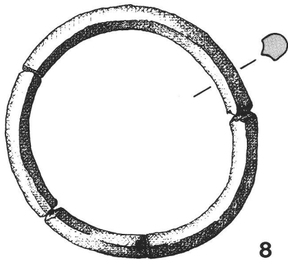
Abb. 4 Totentanz 7 (1984/27). Streufunde (1-6) (1,2 vermutlich aus demselben Grab): 1 lavezimitierender Keramik- becher; 2,3, Teller; 4,5 RS von Töpfen; 6 BS von Krug. Grab 1 (7-10): 7 Bronzearmreif, 8 Lignit- armreif, 9 Becher mit braunrotem metallisierendem Überzug, 10 Bodenfragment eines Sigillata- tellers. Grab 2: 11 Teller. - 7,8 M. 1:1; übrige M. 1:2. Zeichnung M. Wagner.
