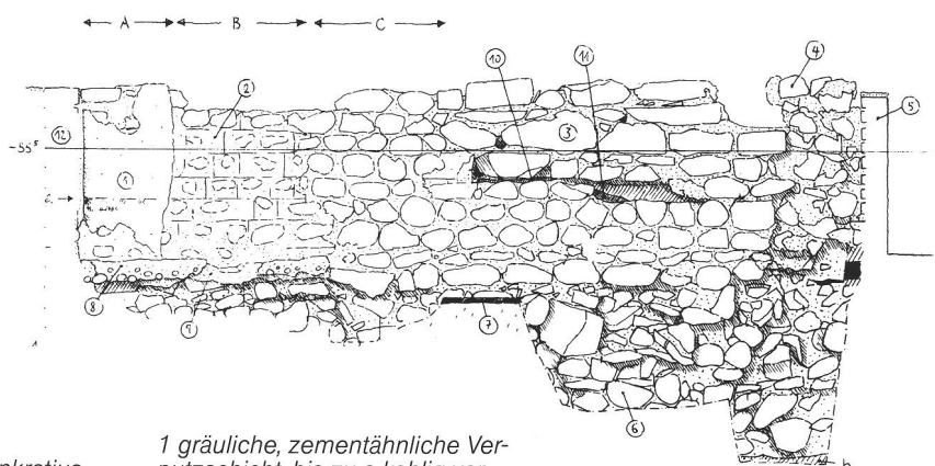
A – C geben verschiedenen präparierten Mauerzustände wieder: A nachrömische Verputzschicht 1 B der darunterliegende römische, steinsichtige Verputz mit Fugenstrich 2 C Mauerbeschaffenheit der römischen Mauer unter der Verputzschicht 2
