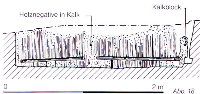
Abb. 18 Kalksumpfrube mit deut- lich sichtbaren Negativen der Holzaukleidung. Zeichnung Johannes Weiss. Une fosse à chaux avec son coffrage en bois. Calcinaio rivestito di legno.
