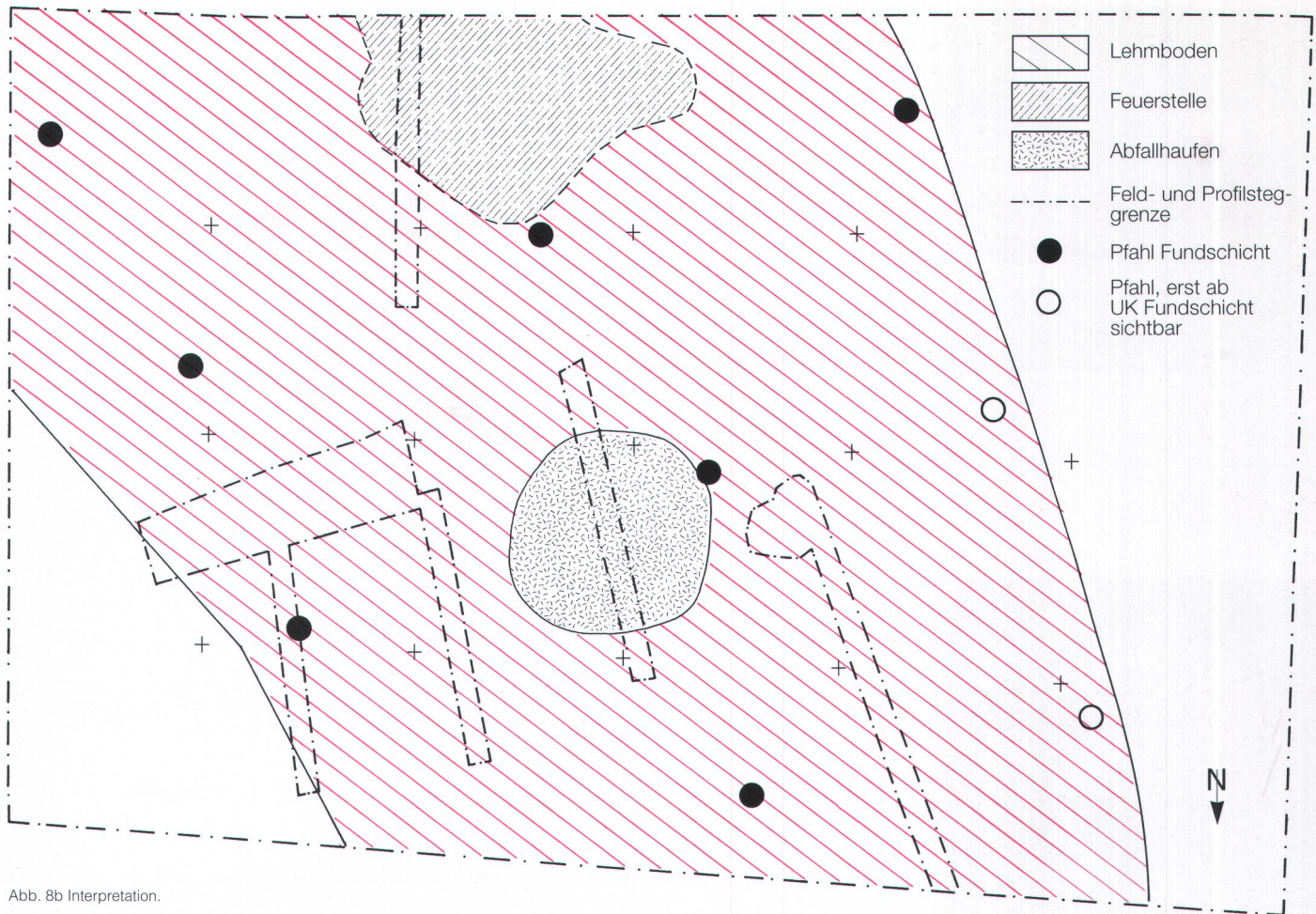
Abb. 8 Ausschnitt des Hauses »Ost« nach Abtrag des Lehm Bodens (vgl. Abb. 5). Der Hausgrundriss misst 4,5 m in der Breite. Der seewärts leicht verrutschte Lehm Boden wird von den Wandpfosten aus Weisstannenh Holz begrenzt. Darunter zeigt sich an gewissen Stellen eine Lage aus dünnen Holzstämmen, die eine Art Rost bilden. Weiter ist die Firstpfostenreihe, ein Abfallhaufen und eine Feuerstelle sichtbar (Foto Kantonsarchäologie Zug/A. Ottiger; Zeichnung S. Nüssli Baltensweiler). Vue partielle de la maison »est« (cf. fig. 5). Le plan au sol du bâtiment mesure 4,5 m de large. La chape d'argile, légèrement déplacée vers le lac, est délimitée par les pieux de parois en sapin blanc. En dessous, on reconnaît par endroits une couche de branches formant une sorte de plancher. On observe en outre une rangée de poteaux de faitage, un amas de déchets et un foyer. Particolare dell'edificio »est«, della larghezza è di 4,5 m (cf. fig. 5). Il suolo di argilla, slittato leggermente verso il lago, è delimitato dai pali di abete che reggevano le pareti. Al di sotto si delinea a tratti una sorta di grata formata da sottili tronchi. Si riconoscono inoltre i pali di calmo, un deposito di rifiuti ed un focolare.
