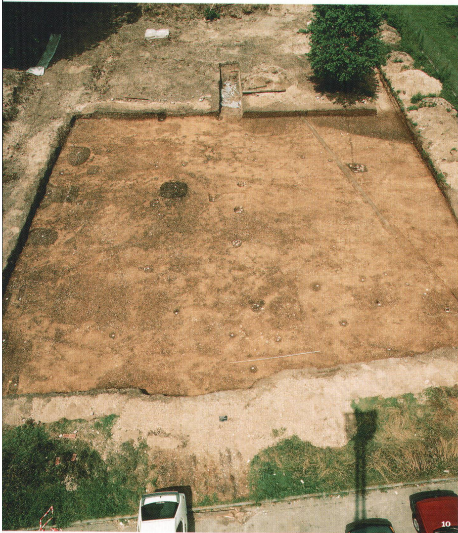
Abb. 10 Sonceboz-Rue Pierre Pertuis, Übersicht über die freigelegte Fläche mit sichtbaren Reihen von Pfostenlöchern und Gruben.
