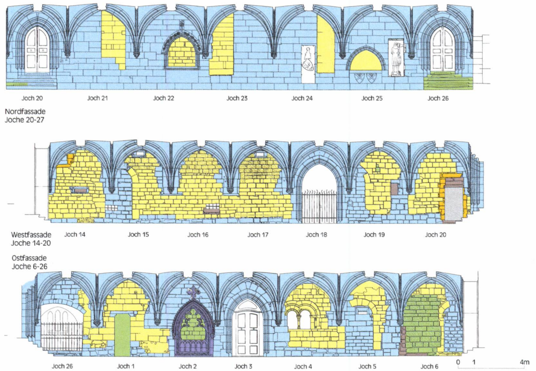
Abb. 4 Aufrisse der Kreuzgangwände. Gelb: aus der romanischen Epoche erhaltene Strukturen. Dunkelgelb: Elemente aus dem 13. Jahrhun- dert. Blau: zum gotischen Neubau gehörende Teile. Violett: während der gotischen Bauphase geschaffenes Nischengrab. Grau: Umbaumas- snahmen des 18. Jahrhunderts. Grün: die aus der Zeit der Renovation von 1903–1913 stammenden Teile.
