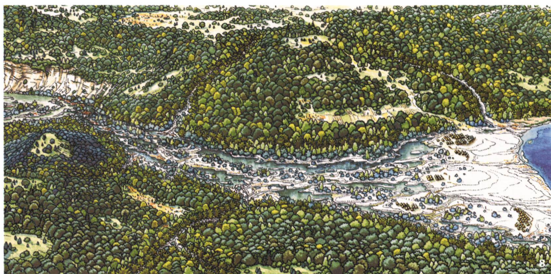
Fig. 8 Occupation de la rade de Genève au Bronze final (vers 1000 av. J.-C.). Plusieurs villages littoraux sont établis sur le banc de sable et d'argile temporairement asséché. Pendant les plus bas niveaux du Léman (environ 3 m plus bas que l'actuel), le Rhône ne s'écoulait plus à Genève, où son cours était réduit à quelques ruisseaux qui se jetaient plus en aval dans l'Arve. Le paysage végétal comprend la plupart des essences présentes aujourd'hui, mais dans des proportions et des situations différentes.
