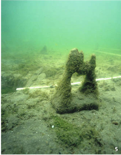
Abb. 5 Prähistorischer Brückenpfahl bei Hurden. Ein Einsinken in den Untergrund wurde dadurch verhindert, dass durch das Loch ein Querbalken gelegt wurde.
