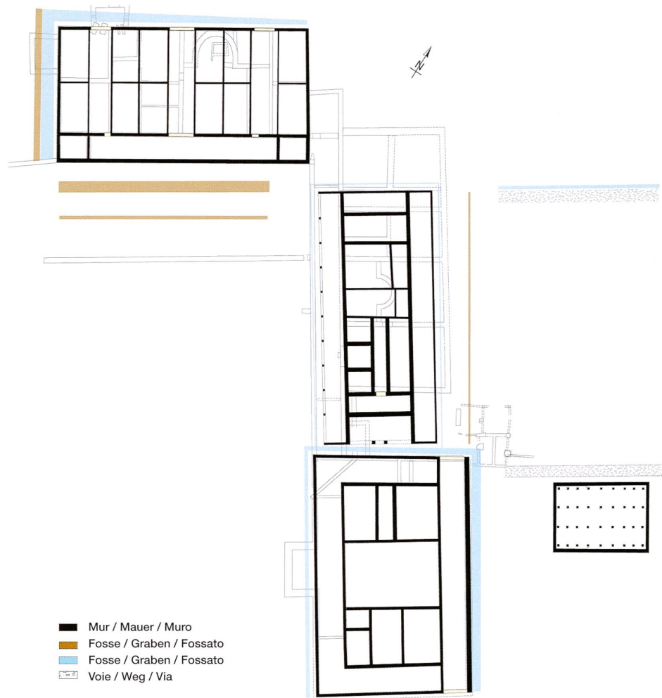
Fig. 27 Vallon – Sur Dompierre. Plan du concept architectural de la période flaviano-trajane.
