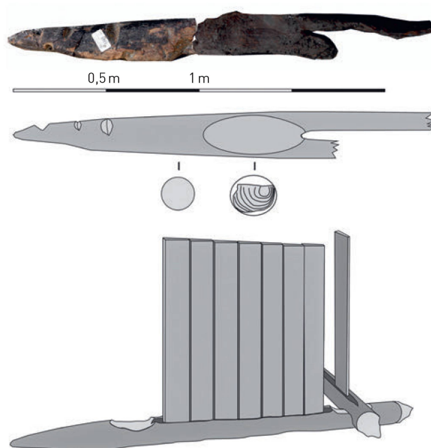
5 Der aussergewöhnliche Fund eines Schwellbalkens mit Längsnut lässt vermuten, dass die Häuser in Immensee nicht aus Flechtwerk mit Lehmbewurf bestanden, sondern aus senkrecht eingesetzten Bohlen.
