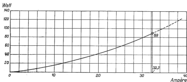
Abbildung 16. Zusätzliche Verluste der Gleichstrommaschine in Abhängigkeit von der Nutzstromstärke.
