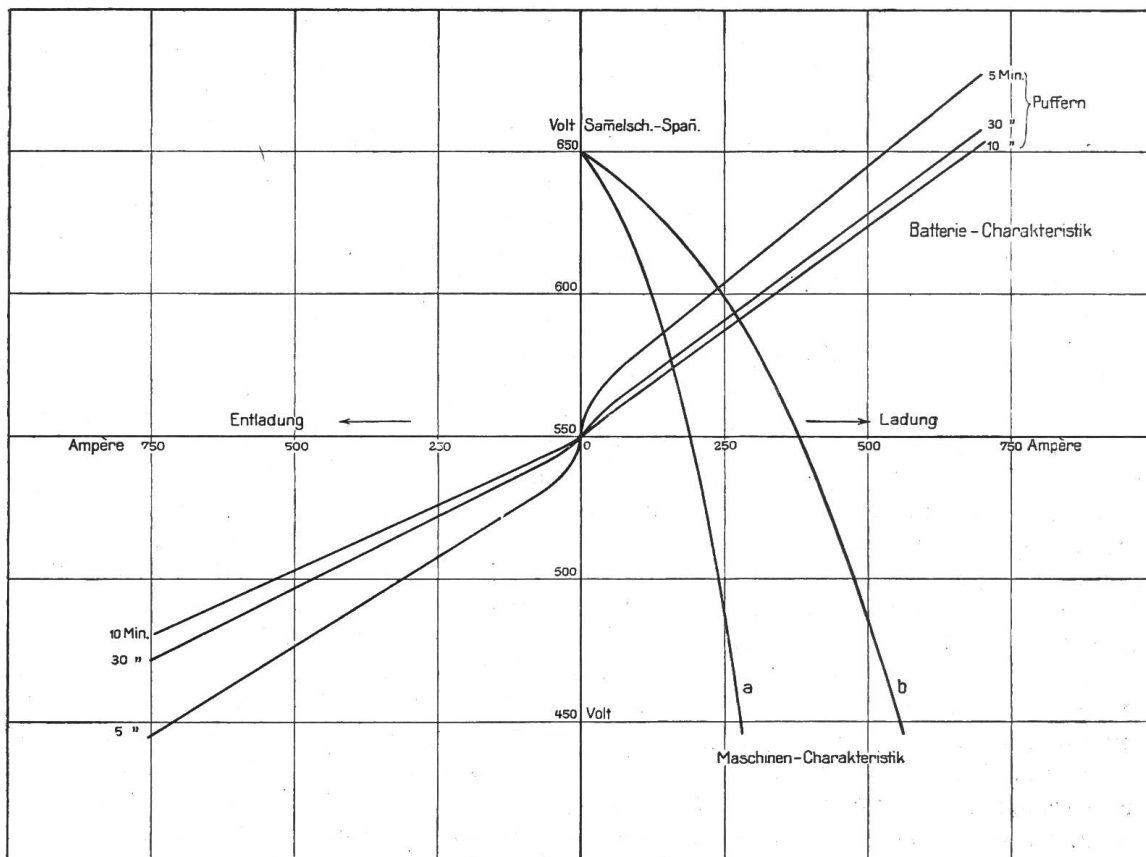
Abbildung 1 a. Kombination der Charakteristiken von Batterie und Maschinen; Gleichstrom-Nebenschluss-Generatoren von 105 KW bei 550 Volt (a wenn eine Maschine, b wenn zwei Maschinen im Betrieb); Pufferbatterie von 268 Elementen von 407 Ampèrestunden.
