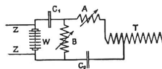
Abbildung 7: Schaltung bei Löschfunken.
