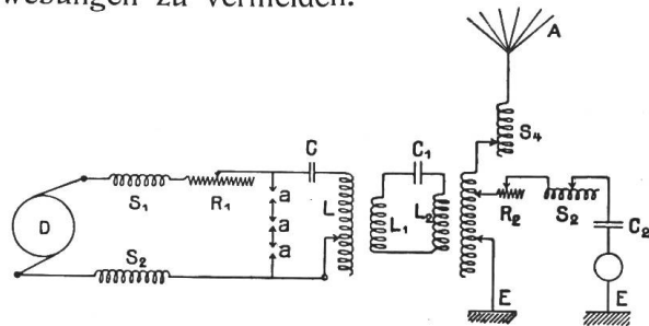
Abbildung 26. Radiotelephonie nach Colin-Jeance. D = Dynamo, a = Lichtbogen, A = Antenne, E = Erde.
