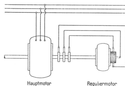
Abb. 7. Drehstrom-Hüttenmaschinenantrieb nach dem Reguliersystem mit Drehstromkommutator-Hintermotor nach Krämer.
