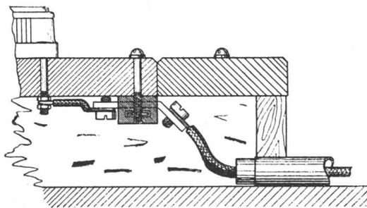
Abb. 7. Extra-Verteilungsklemme, bei welcher die Kontrolle der Anschlussleitung handgreiflich vorgenommen werden kann, nach Abnahme einer Deckplatte. Auch hier sind die Klemmen hinter der Tafel unkontrollierbar
