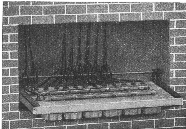
Abb. 8. Verteilungstafel mit Schalttafelelementen, zur Kontrolle der Rückseite scharnierartig umgelegt (Klapptafel).
