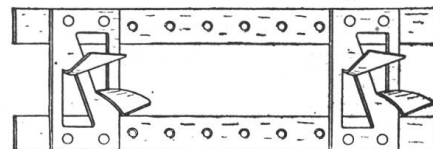
Abb. 20. Dübelrahmen für ältere Universalsicherungen.
