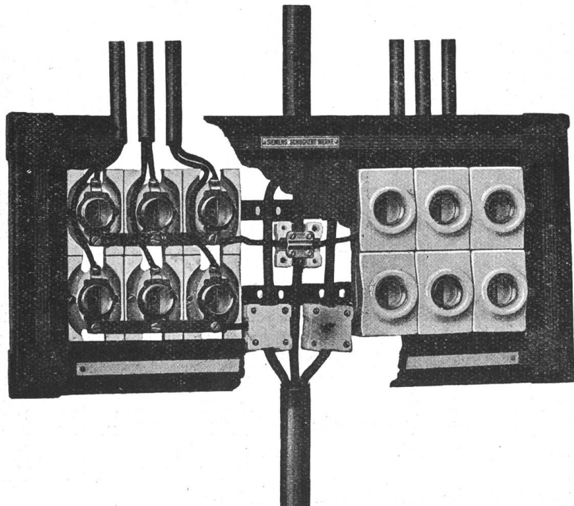
Abb. 37. Dreileitergruppe mit zweipoligen Abzweigungen und durchgehender Steigleitung in der Mitte.
