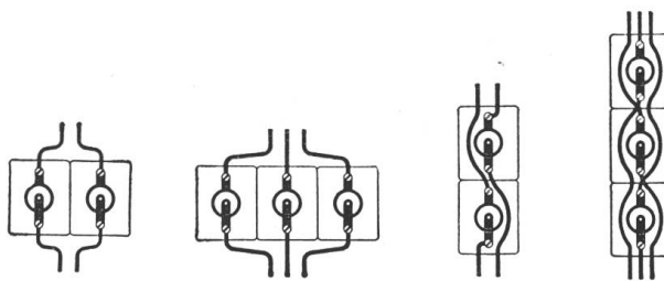
Abb. 15. Schemata für Uzed-Einzelsicherungen.
