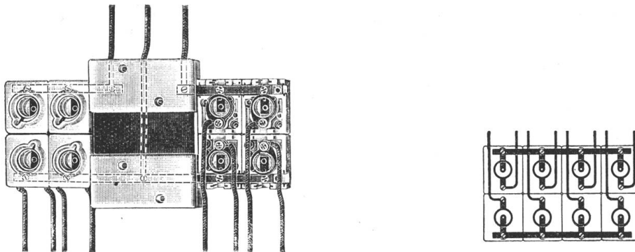
Abb. 13. Universalsicherungen mit Sammelschienen samt Leitungen auf der Vorderseite.
