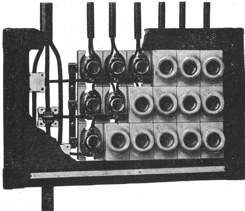
Abb. 36. Dreileitergruppe mit dreipoligen Abzwegsicherungen und seitlichem Anschluss.
