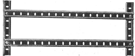
Abb. 23. Fertiges, aus Hohlchienen gebildetes Befestigungsgestell, als Unterlage für eine Uzed-Gruppe.
