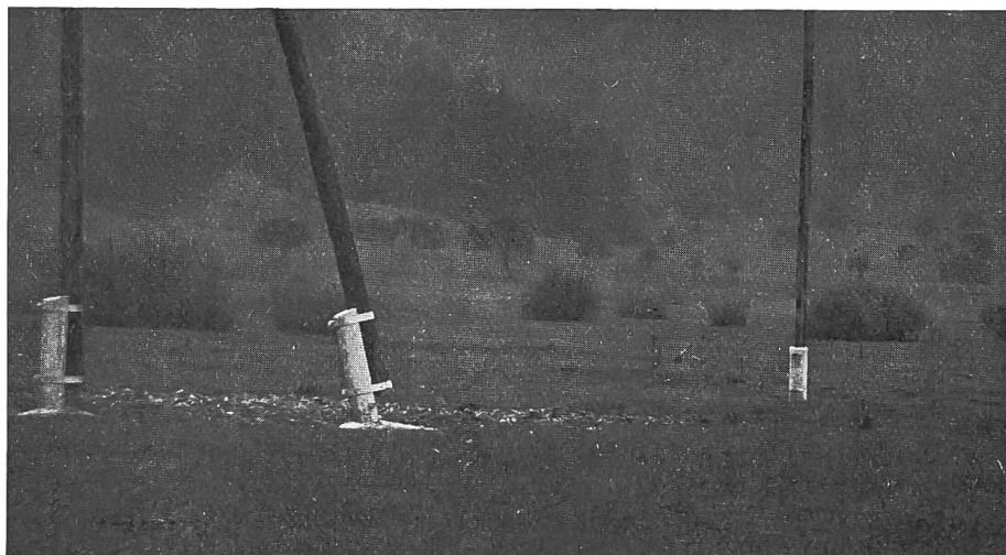
Fig. 9. Leitung auf „Universalsöckeln“ durch Sumpfgebiet.
