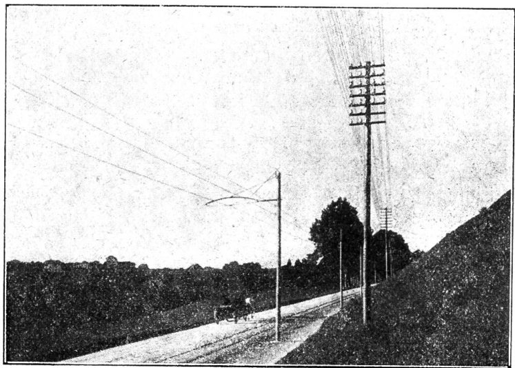
Abb. 12. Fahrdrathträger und Telefonleitung sind beide richtigerweise am aufsteigenden Rand der Strasse aufgestellt; dagegen hätte das Trottoir an den Aussenrand gehört. Durch die schwache Biegung des Auslegers gewinnt der Fahrdrathträger an Gefälligkeit.
