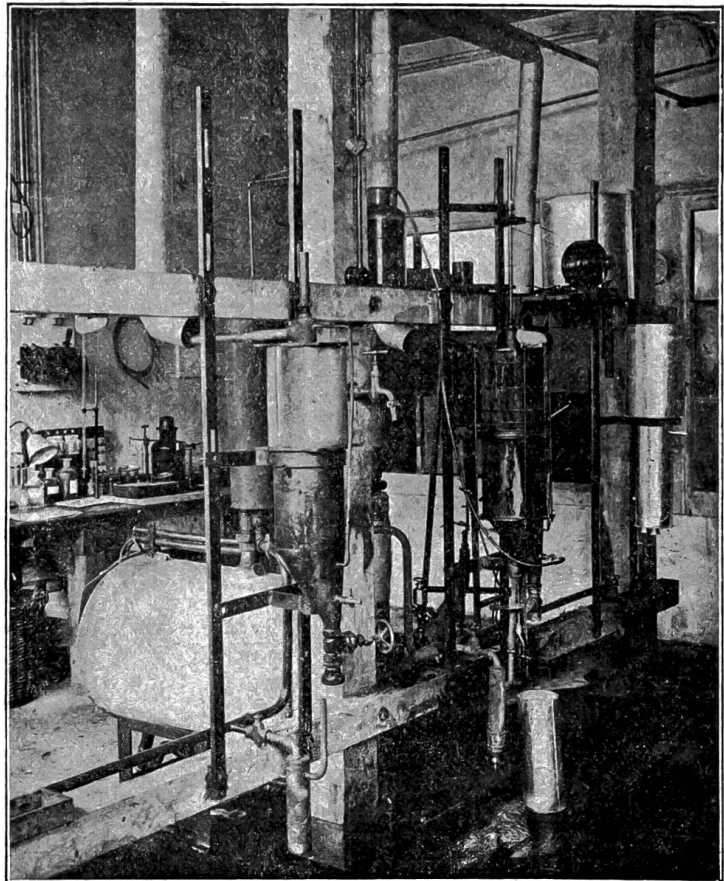
Fig. 3. Laboratorium der A.-G. Kümmler & Matter für Eindampfversuche.
