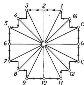
Fig. 13 a - c Zweiphasige Schleifenwicklung mit verkürztem Schritt, nach Lamme (Arnold, W. T. Bd. 3, 1. Aufl. S. 121).
