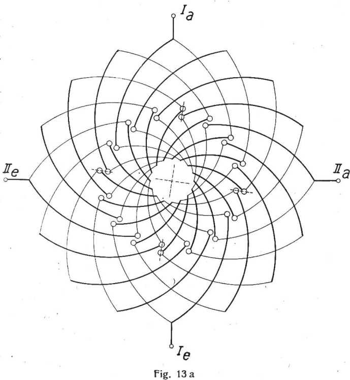
Fig. 13 a - c Zweiphasige Schleifenwicklung mit verkürztem Schritt, nach Lamme (Arnold, W. T. Bd. 3, 1. Aufl. S. 121).
