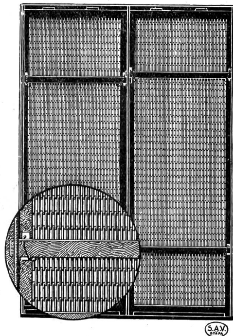
Fig. 4 Gliederband-Filter (Spezialkonstruktion).
