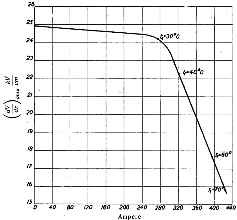
Fig. 16 Maximaler Spannungsgradient in Funktion des Leiterstromes von Kabel No. 3 bei Gleichstrom. Bei homogener Spannungsverteilung beträgt der Gradient 15 KV/cm. t_1 bedeutet die Leitertemperatur, die Raumtemperatur ist 7^\circ\text{C} . Bei t_1 = 30, 40 und 50^\circ\text{C} liegt der maximale Gradient an der Leiteroberfläche entsprechend einem Radius r_1 = 0,65 cm. Der Mantelradius beträgt r_2 = 1,65 cm. Bei t_1 = 70^\circ\text{C} liegt der maximale Gradient bei r = 0,85 cm.
