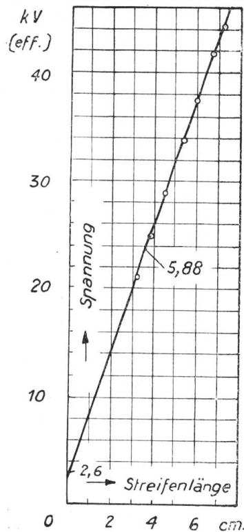
Fig. 5. Hartpapierrohr \epsilon_2 = 4.5 , 4,5/6 cm Durchm. E_{st} = 5,88 kV/cm. \zeta_{st} = 11,8 kV/cm.
