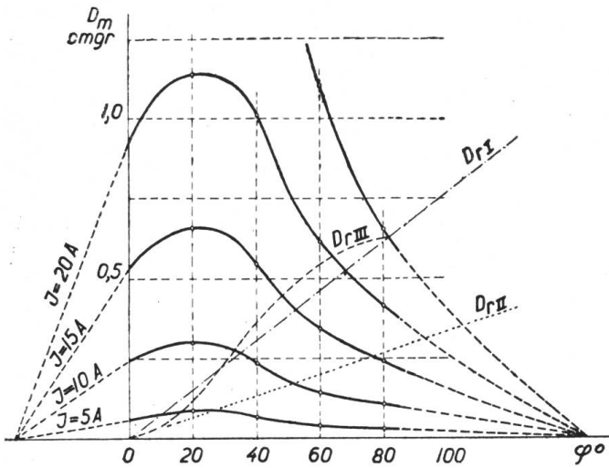
Fig. 1. Elektrisches und mechanisches Drehmoment in Funktion des Skalenwinkels.
