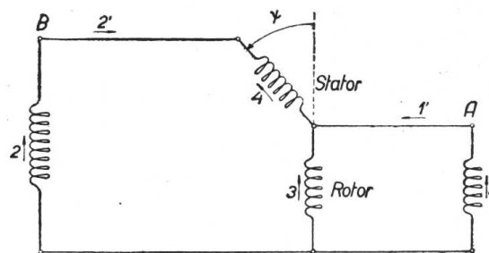
Fig. 7. Prinzipielles Einbauschema eines Induktionsreglers ins Netz.
