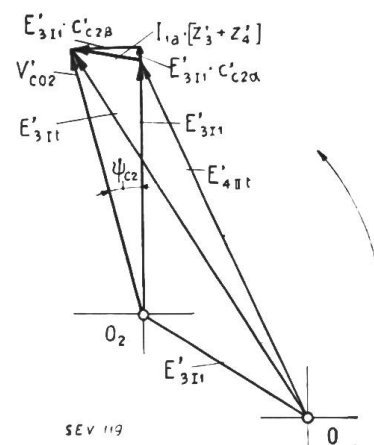
Fig. 12. Leerlaufdiagramm der treibenden Spannung im Kaskadenkreis bei sekundärer Spannung.
