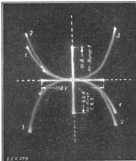
Fig. 14. Widerstands-Oscillogramme eines Silitringes mit 200 \Omega Nennwert, samt Eichwerten der Spannungs- und Stromachse. Kurven 1 bis 3: Drei Aufnahmen bei annähernd derselben Spannung. Für Kurve 3 Anschluss der Spannungs-Ablenkplatten vertauscht.
