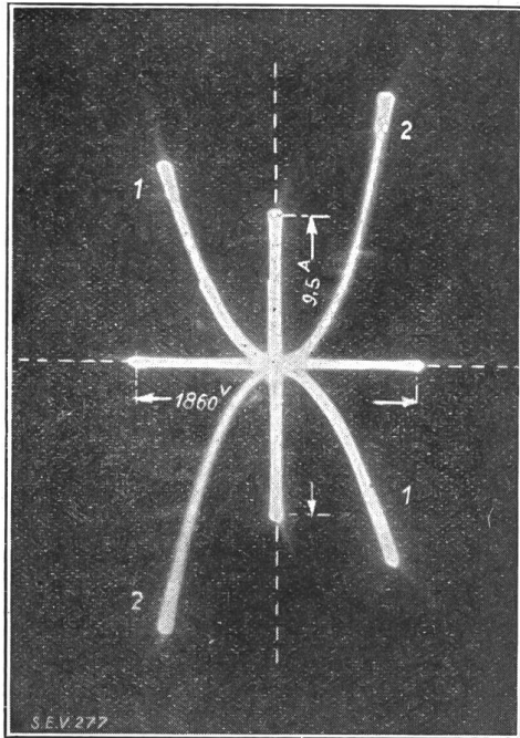
Fig. 12. Widerstands-Oscillogramme eines Silitstabs mit 700 \Omega Nennwert, bei zwei verschiedenen Spannungen mit vertauschtem Anschluss der Spannungs-Ablenkplatten aufgenommen (Kurven 1 und 2), samt zugehörigen Eichwerten der Spannungs- und Stromachse.
