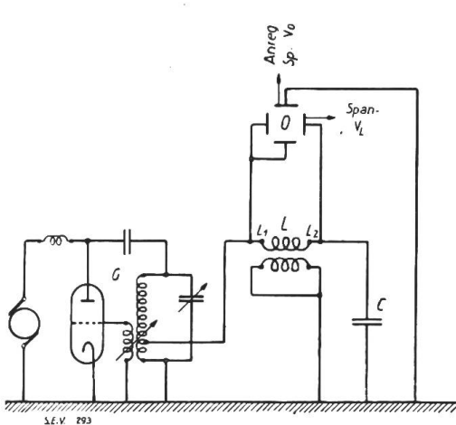
Fig. 29. Anordnung zur Resonanzspannungsmessung.
