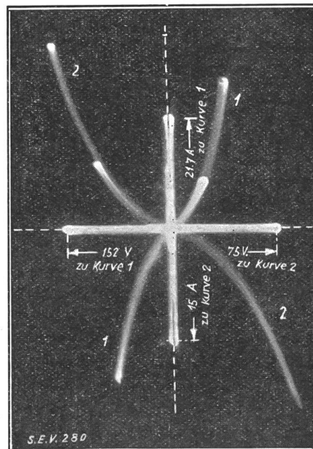
Fig. 15. Widerstands-Oscillogramme eines Silitringes mit 5 \Omega Nennwert, samt Eichwerten der Spannungs- und Stromachse. Anschluss der Spannungs-Ablenkplatten zwischen den Aufnahmen 1 und 2 vertauscht.
