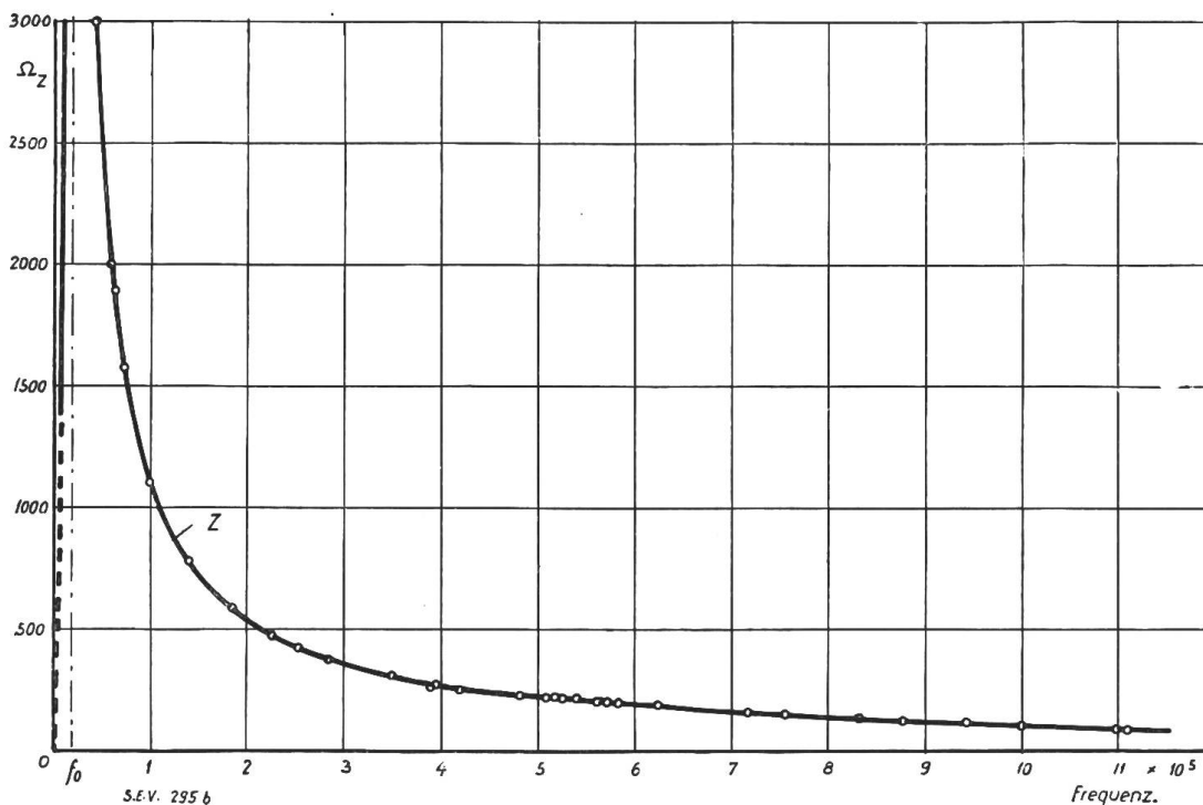
Fig. 30 b. Impedanzkurve Z desselben Stromwandlers wie Fig. 30 a im Frequenzbereich bis ca. 10^6 Perioden.
