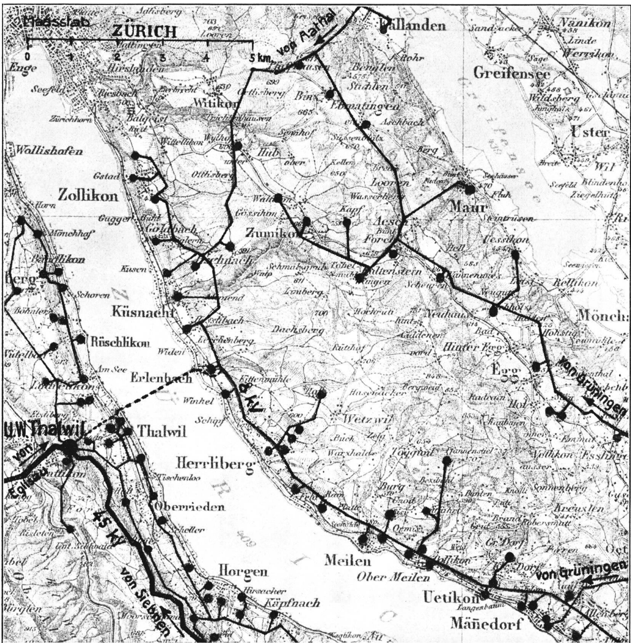
Fig. 1. Uebersichtsplan der Verteilungsanlagen am unteren Zürichsee. (Reproduziert mit Bewilligung der Eidg. Landestopographie vom 8. Nov. 1928.)
