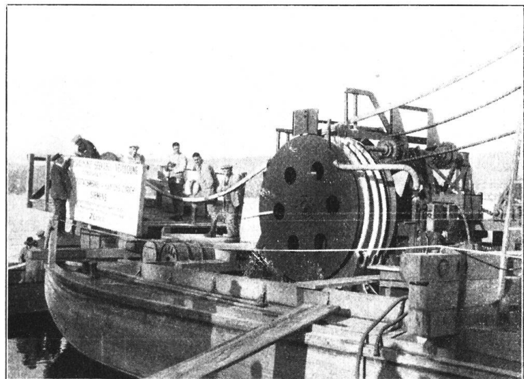
Fig. 6. Kabelverlegungsmaschine.
