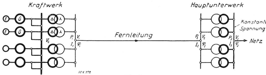
Fig. 3. Einpoliges Uebersichtsschema der Uebertragung ohne Blindlastkompensation.
