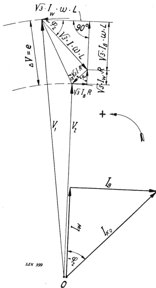
Fig. 4. Vektordiagramm für Strom und Spannung, den Spannungsabfall einer Leitung darstellend.
