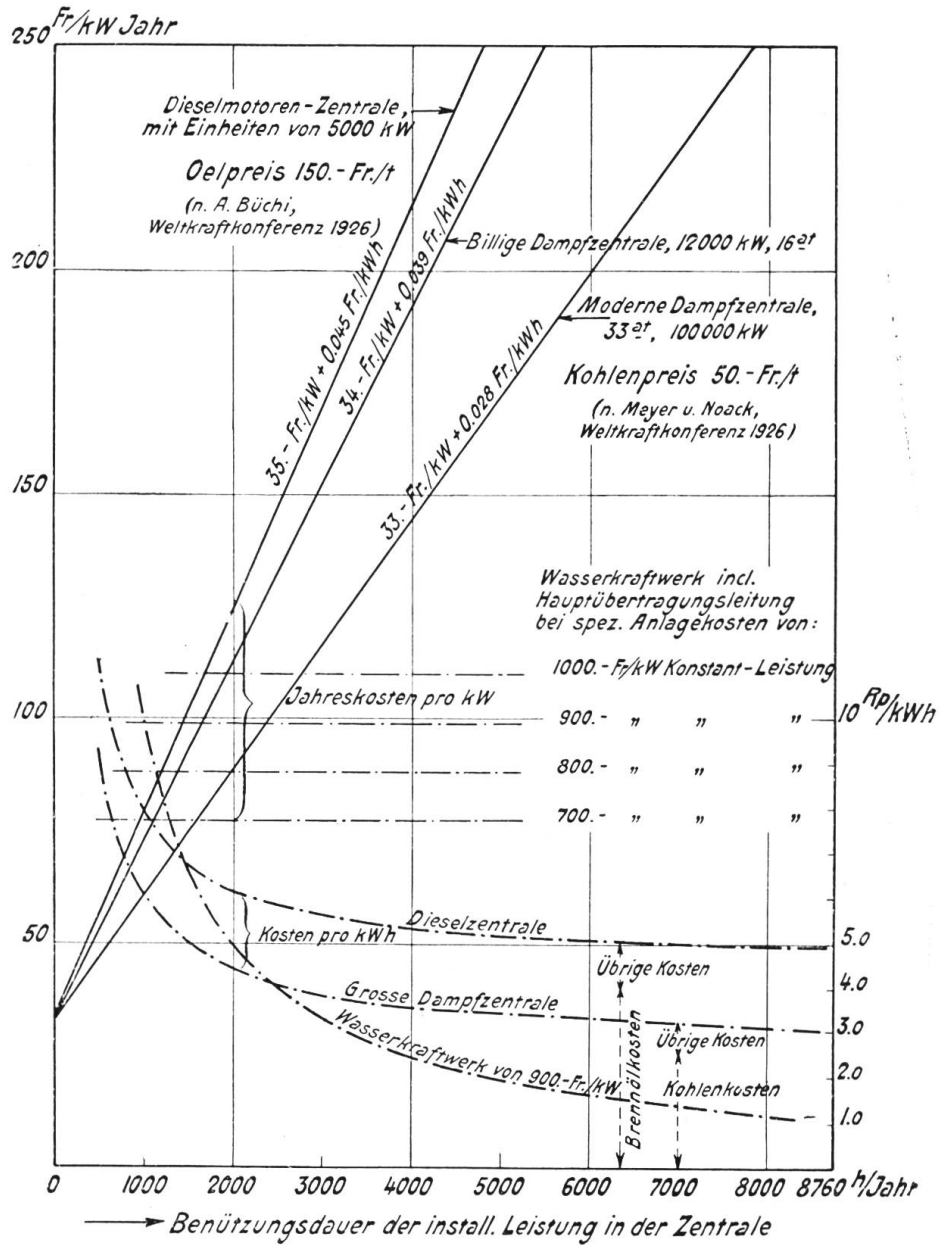
Fig. 3. Vergleich der Jahreskosten von Wasser- und Wärmekraftwerken.
