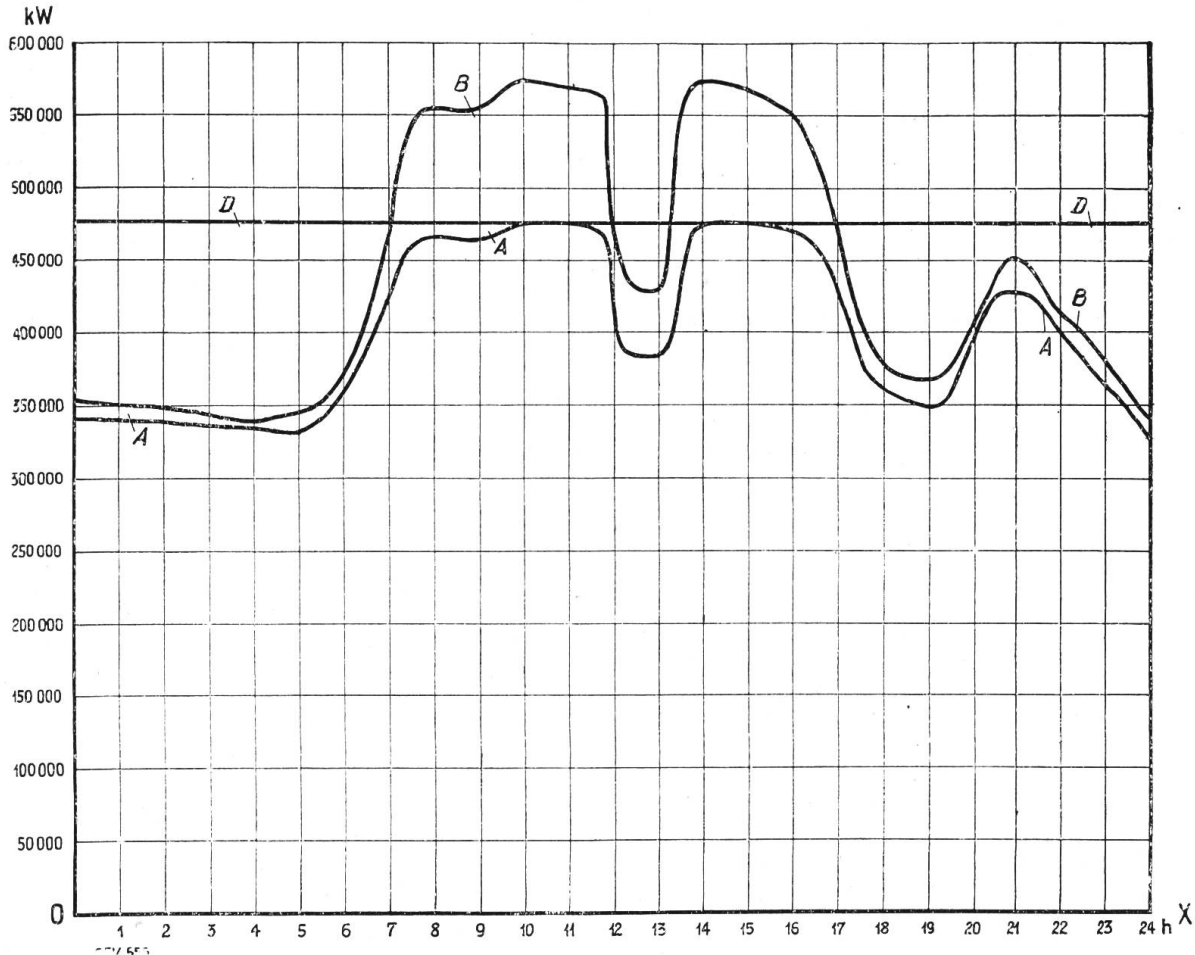
Verlauf der wirklichen Gesamtbelastungen am 16. Mai 1928. Diagramme journalier de la production totale le 16 mai 1928.
