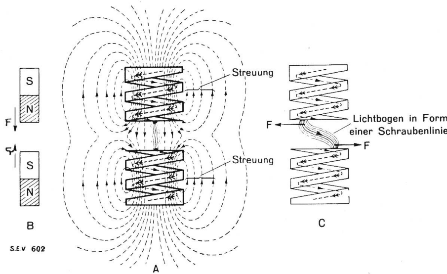
Fig. 11. Schematische Erklärung der Eigenblasung bei Solenoidkontakten. Die Streufelder bewirken eine Ausblasung des Lichtbogens in Form einer Schraubenlinie.
