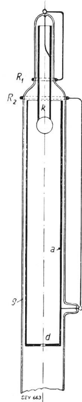
Fig. 2. Entladerohr nach Busch (aus A.f.E., Bd. 18, S. 592).
