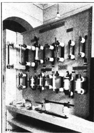
Fig. 7. Trenner_und Trennsicherungen.
