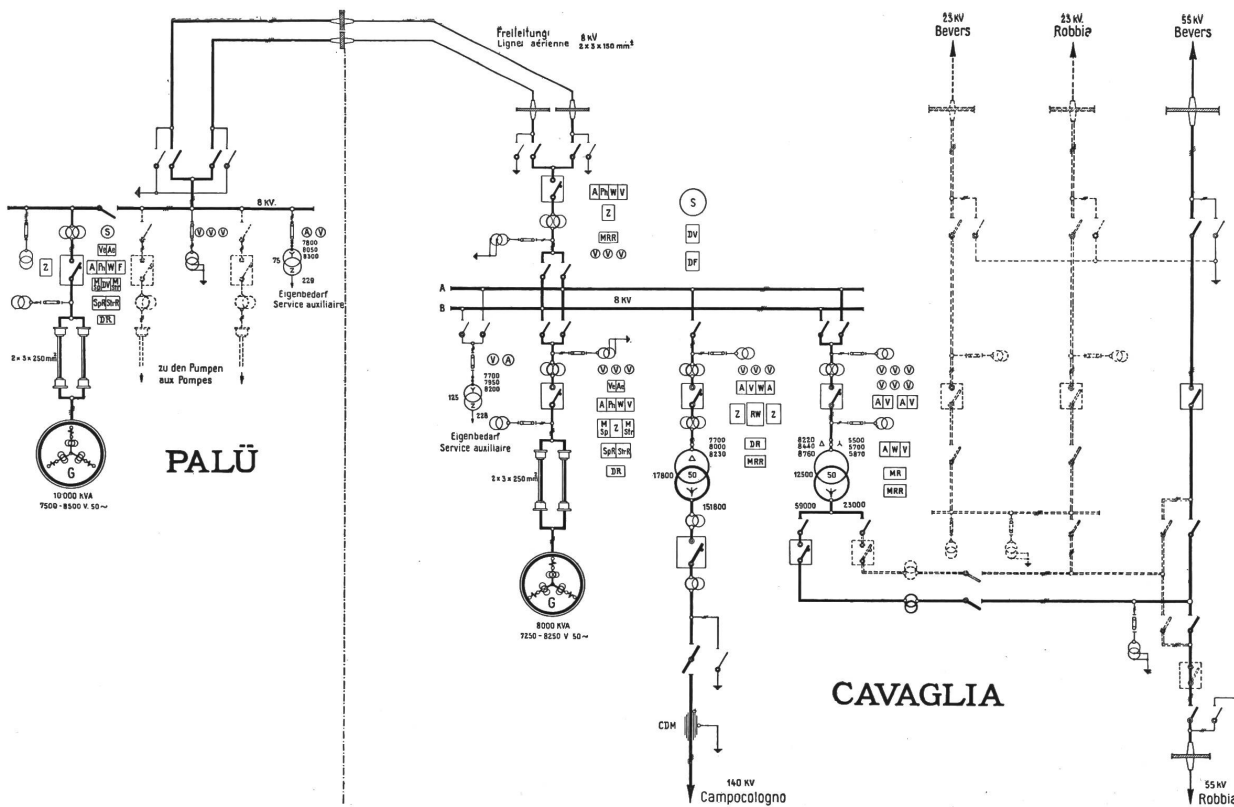
Fig. 10. Kraftwerke Palù-Cavaglia. Schaltungsschema.
