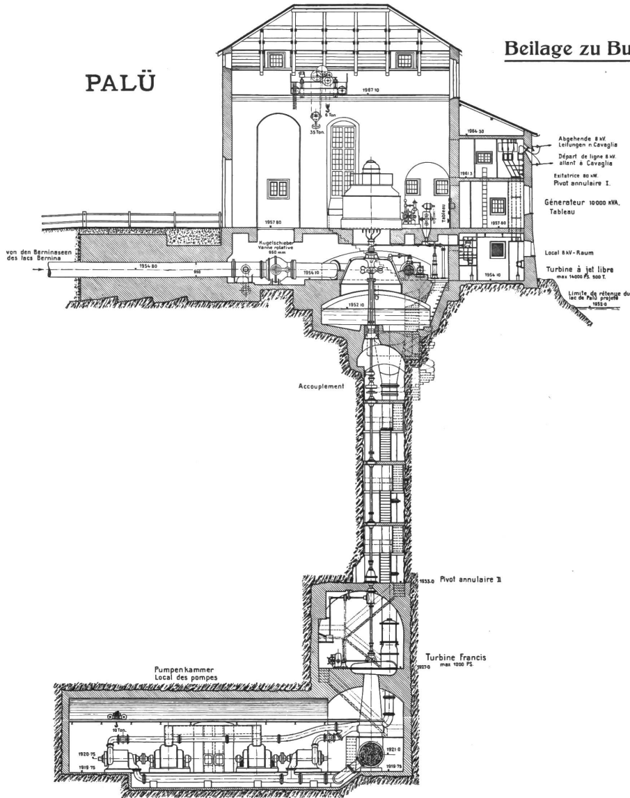
Fig. 6. Kraftwerk Palü. Schnitt durch die Maschinenhausanlage.
